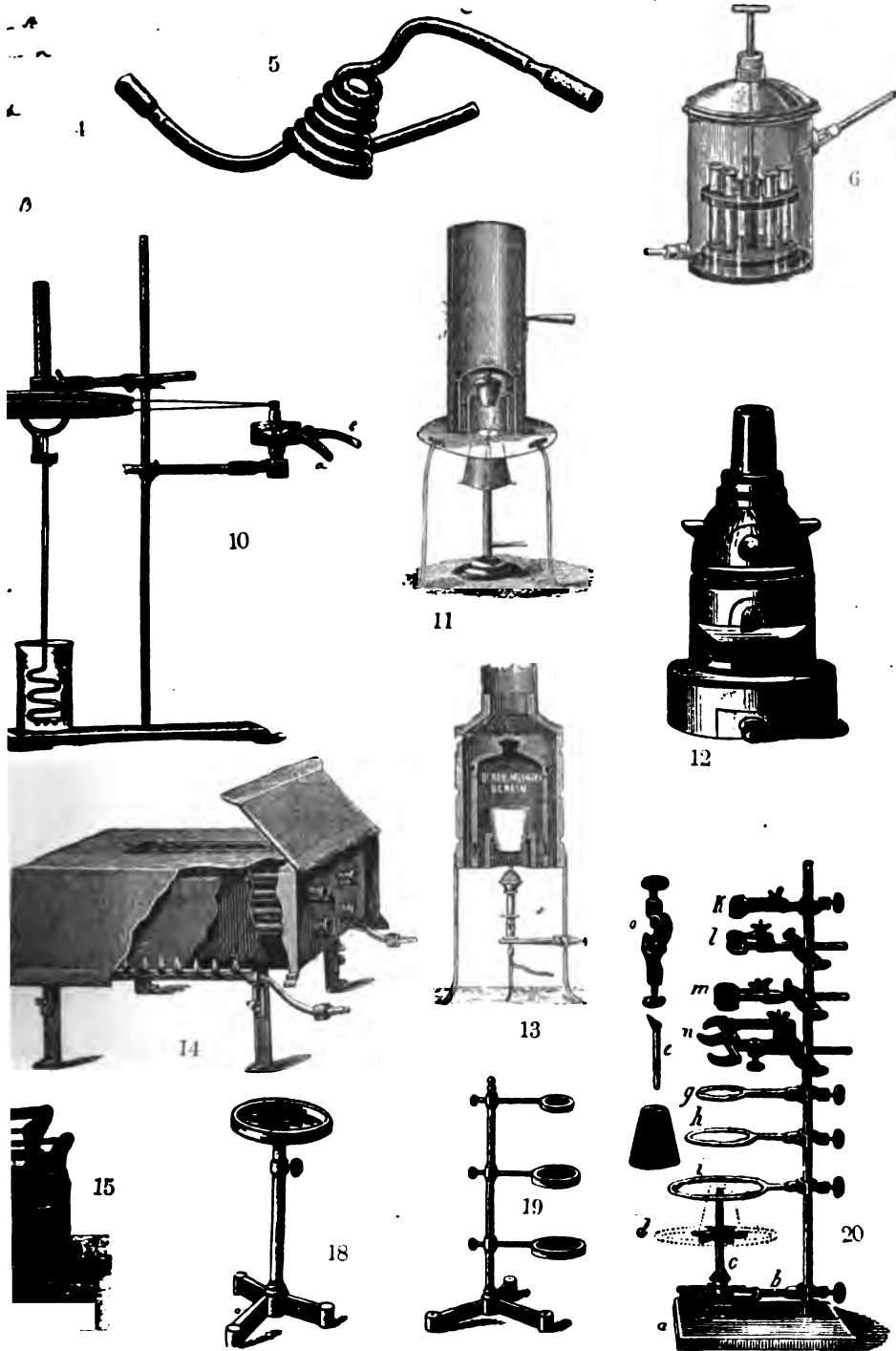
для перегривания пара. 6. Прибор Горбова и Кесслера для перегонки под уменьшенным давлением Рабе. 11. Печь Гемпеля. 12. Шамотовая печь калильная. 13. Печь Мюнке. 14. Печь Лотара для сушки газов. 18. Подставка. 19. Штатив для вронков. 20. Универсальный штатив Бунзена.
